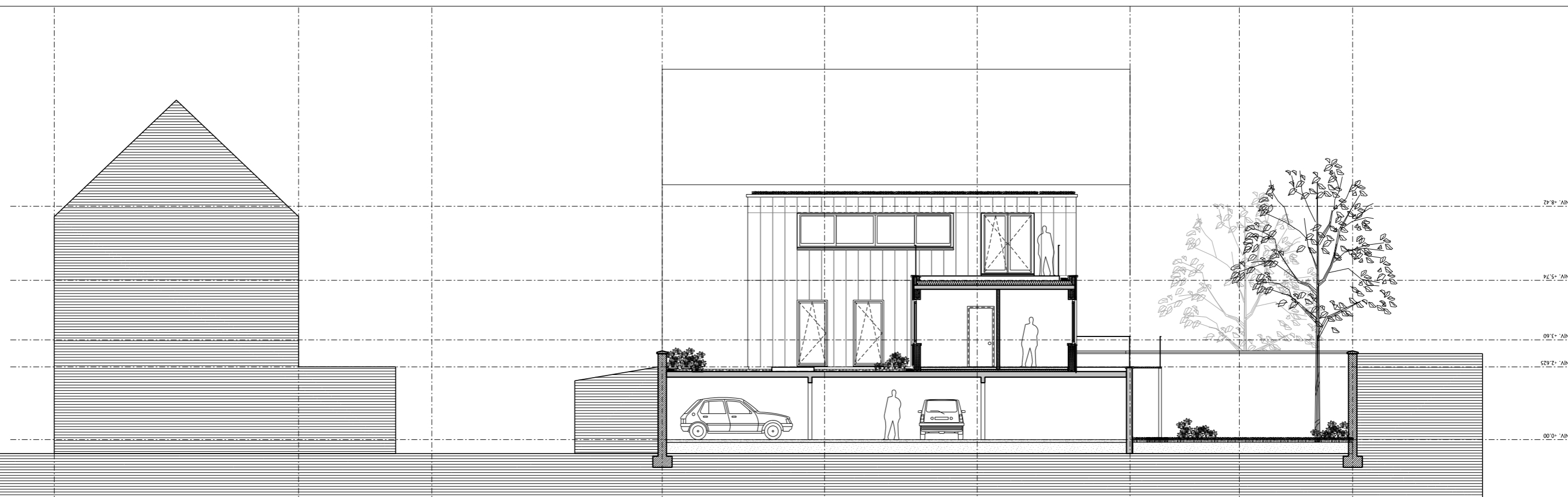
COUPE BB
