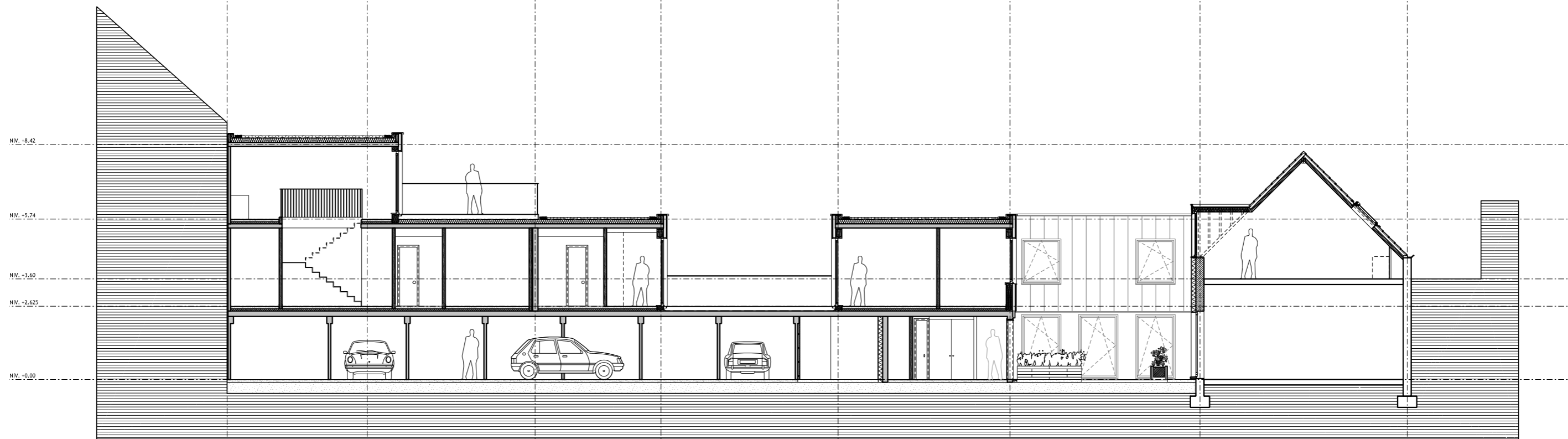
COUPE AA
